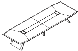
ED78 W4800•D1600•H760(mm)
