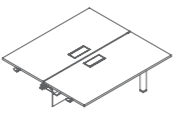
DE636-5.12K/DE626-5.12K W1200•D1212•H750 DE636-5.14K/DE626-5.14K W1400•D1412•H750 DE636-5.15K/DE626-5.15K W1500•D1412•H750 DE636-5.16K/DE626-5.16K W1600•D1412•H750
