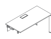
DE637-5.12K/DE627-5.12K W1200•D600•H750 DE637-5.14K/DE627-5.14K W1400•D700•H750 DE637-5.15K/DE627-5.15K W1500•D700•H750 DE637-5.16K/DE627-5.16K W1600•D700•H750
