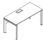
DE67-5.12K W1200•D600•H750 DE67-5.14K W1400•D700•H750 DE67-5.15K W1500•D700•H750 DE67-5.16K W1600•D700•H750
