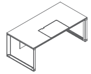
DE86-5.18 W1800•D900•H750 DE86-5.20 W2000•D1000•H750 DE86-5.22 W2200•D1000•H750
