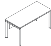
DE85-5.12 W1200•D600•H750 DE85-5.14 W1400•D700•H750 DE85-5.15 W1500•D700•H750 DE85-5.16 W1600•D800•H750 DE85-5.18 W1800•D900•H750
