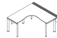
DE60(L/R)-5.14F W1400•D1530•H750 DE60(L/R)-5.15F W1500•D1630•H750 DE60(L/R)-5.16F W1600•D1730•H750
