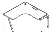
DN62BL/R W1456•D1428•H750(mm) W1556•D1528•H750(mm) W1656•D1628•H750(mm)
