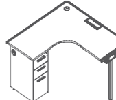
DN62BL/R W1456•D1428•H750(mm) W1556•D1528•H750(mm) W1656•D1628•H750(mm)
