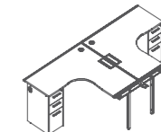
DN63A W1428•D2828•H750(mm) W1528•D3028•H750(mm) W1628•D3228•H750(mm)
