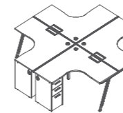
DN64 W2828•D2828•H750(mm) W3028•D3028•H750(mm) W3228•D3228•H750(mm)
