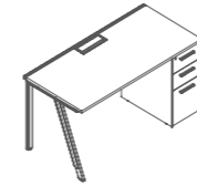
DN60 W1200•D628•H750(mm) W1400•D728•H750(mm) W1500•D728•H750(mm) W1600•D728•H750(mm)
