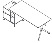
EP83 W2150*D900*H750(mm) W2350*D900*H750(mm)
