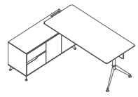
EP81/EP82 W1950*D1850*H750(mm) W2150*D1850*H750(mm) W2350*D1850*H750(mm)
