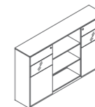
E905-2 W1967*D400*H1201(mm)
