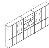
E99-2 W4364*D400*H2005(mm)
