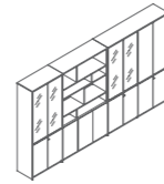
E98R-2 W3579*D400*H2005(mm)
